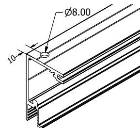
MECANIZADO PARA PERFIL 1120 FIJO LATERAL PARA AUTOPORTANTE.
