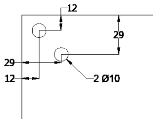
MECANIZADO PARA VIDRIO FIJO LATERAL PARA USAR LA PIEZA CORNER 40.115000.04.
