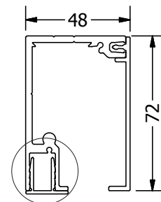
1118 GUÍA FIJO EPROM70 / ELEVA700 DETALLE COLOCACIÓN PERFIL CONTINUACIÓN VIDRIO FIJO.
