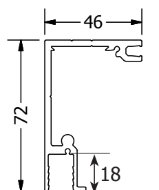
1118 GUÍA FIJO EPROM70 / ELEVA700
