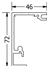
1119 GUÍA EPROM70 / ELEVA700
